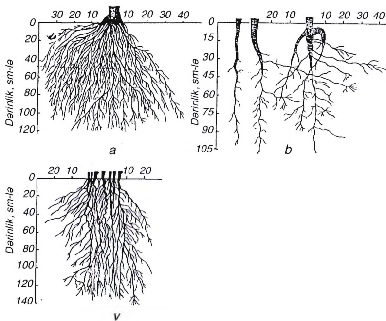
5-ci şəkil. Qrup suları dayazda yerləşən şəraitdə qarğıdalı (a) və pambıq (b, v) bitkilərinin kök sistemi.
