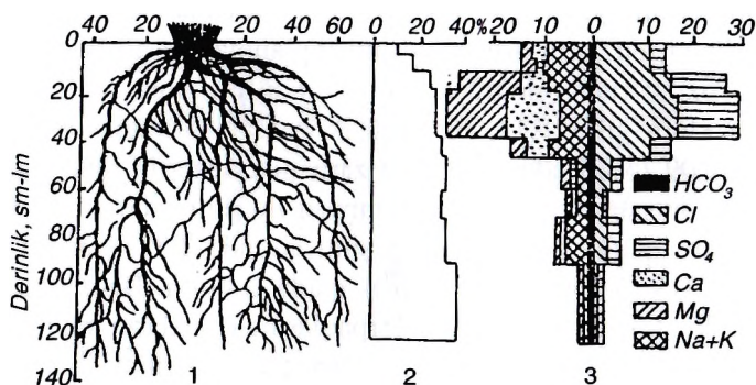
7-ci şəkil. Şovitsa yovşanının kök sistemi (1), torpağın nəmlik (2) və duzluluq (3) profilləri.
