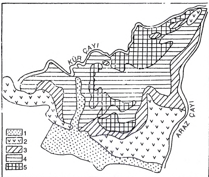
3-cü şəkil. Mil düzü torpaqlarında düz profillərinin tipləri xəritəsi (M.R.Abdüvəv, 1966-cı il). Şərti işarələrin izahı əsərin... 21-22-ci səhifələrində verilir
