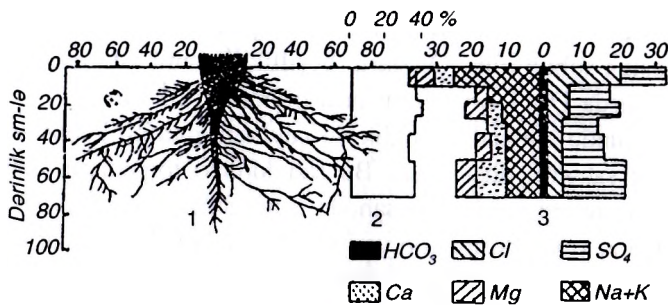
6-cı şəkil. Şovitsa yovşanın kök sistemi (1), torpağın nəmlik (2) və duzluluq (3) profilləri.
