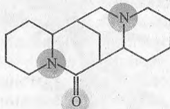
афиллин
