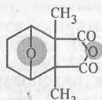
кантаридин
