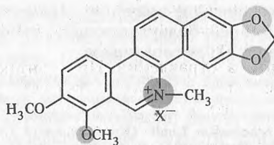
хелеритрин
