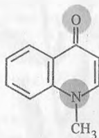
ЭХИНОПСИН
