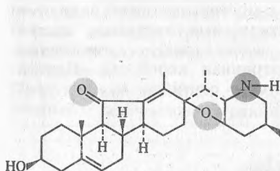
йервин
