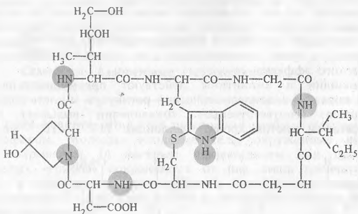
аманин
