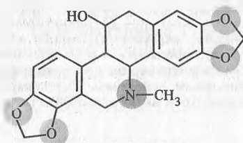
хелидонин
