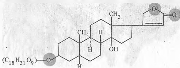
ДИГИТОКСИН
