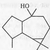
ледол
