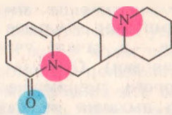
термопсин
