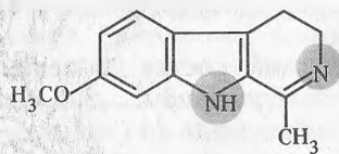
гармалин
