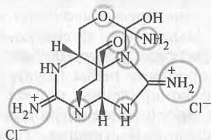
сакситоксин
