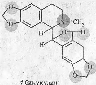
d-бикукулин
