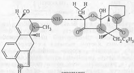
эрготамин
