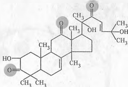
элатерин А
