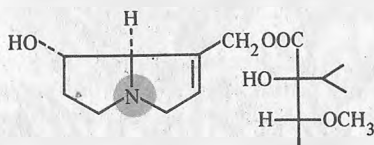
гелиотрин
