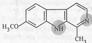
гармин
