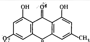
франгулин
