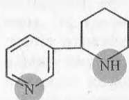
анабазин
