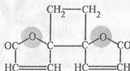
анемонин
