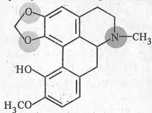
бульбокапнин
