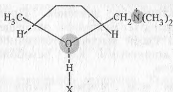
мускарин
