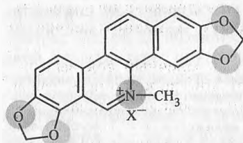
сангвинарин
