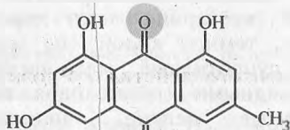
франгулаэмодин
