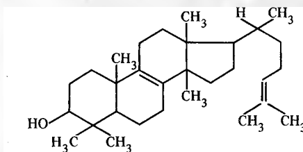
эуфол
