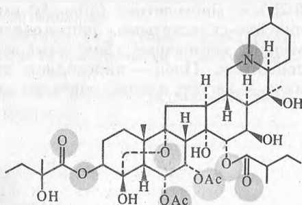
протовератрин А
