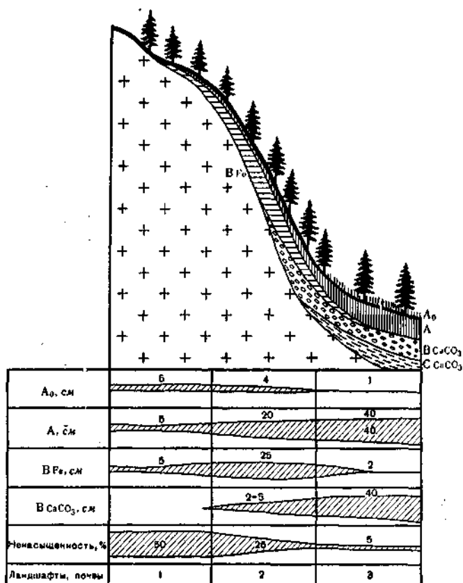
Рис. 24. Почвенно-геохимическое сопряжение в поясе еловых лесов Центрального Тянь-Шаня (По Глазовской, 1968):
