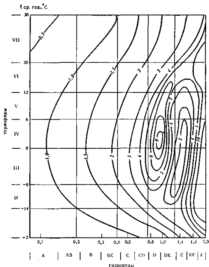
Рис. 4. Содержание гумуса в слое 0—20 см в главных типах почв мира в связи с гидротермическими условиями, % (по В. Р. Волобуеву, 1963)
