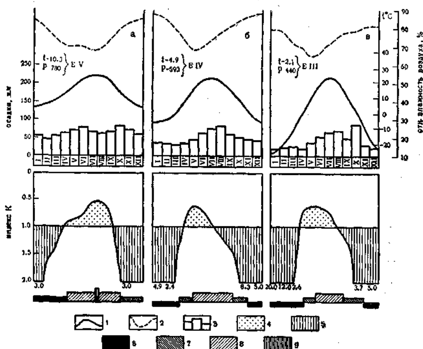
Рис. 96. Гидротермические условия в районах распространения:
