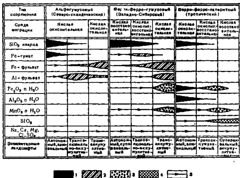
Рис. 21. Типы почвенно-геохимических сопряжений гумидных областей: 1 — остаточная относительная аккумуляция. Геохимические барьеры; 2 — минерализация органической составляющей органо-минеральных комплексов; 3 — окислительные; 4 — биологические; 5 — направление движения веществ
