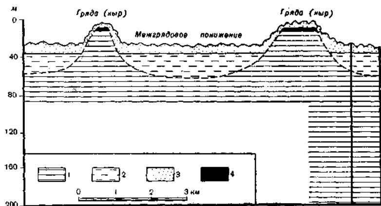
Рис. 62. Условия залегания ископаемых почв на останцах (кырах) плиоценовой аллювиальной равнины (Юго-Восточные Каракумы): 1 — заунгузская свита, 2 — древний аллювий Пра-Амударьи; 3 — золотые пески; 4 — ископаемая почва
