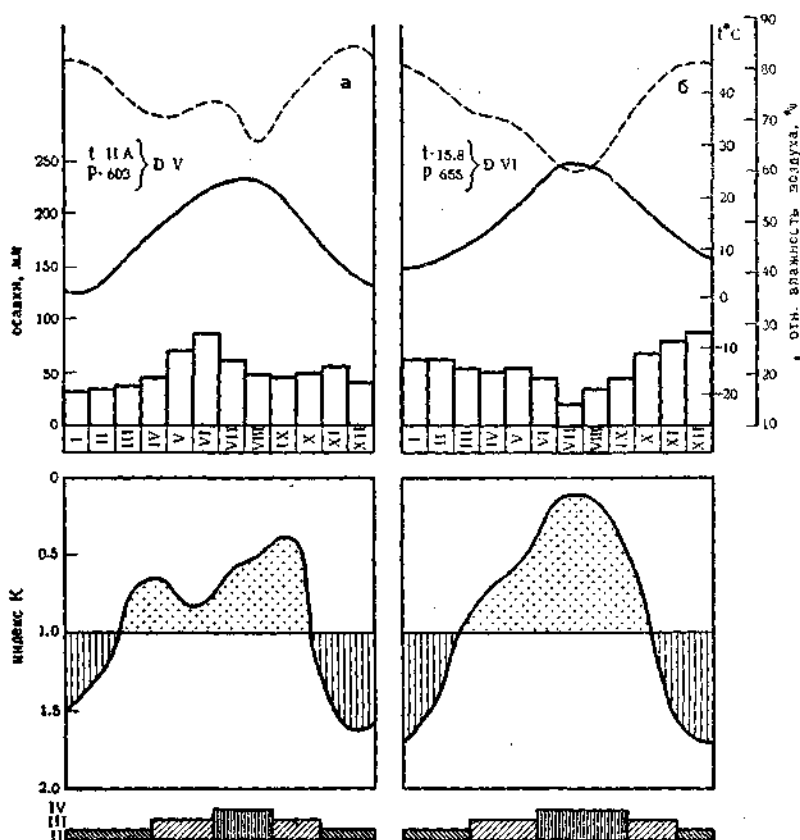
Рис. 41. Гидротермические условия в районах распространения: а — коричневых почв и смольниц; б — коричневых почв Средиземно- морской Европы. Усл. знаки см. рис. 36
