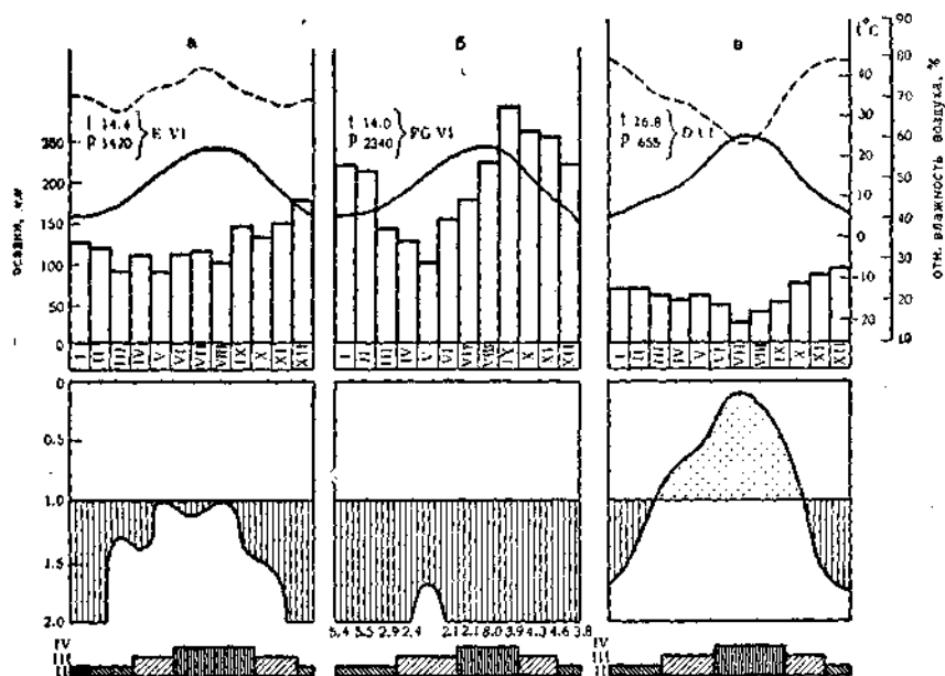
Рис. 43. Гидротермические условия в районах распространения в Закавказье:
