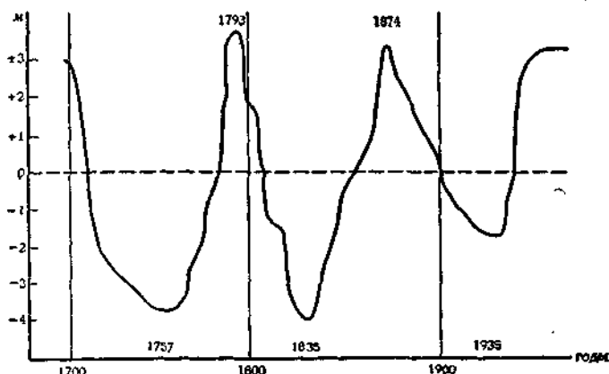
Рис. 16. Колебания уровня озер Западной Сибири за исторический период (по А. В. Шнитникову, 1957)
