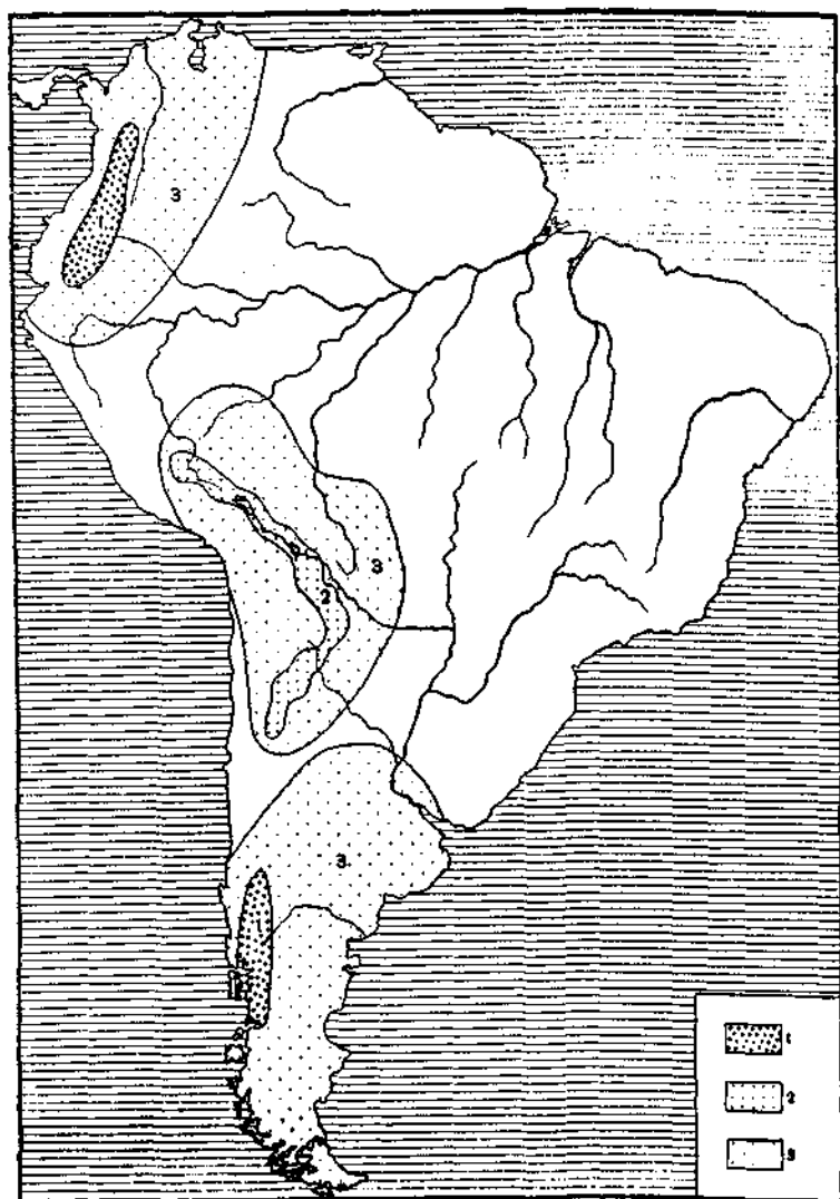
Рис. 69. Распространение вулканических пеплов в Южной Америке: 1 — ландшафты с выветренным вулканическим пеплом; 2 — ландшафты с невыветренным пеплом; 3 — ландшафты со слабыми пеплопадами
