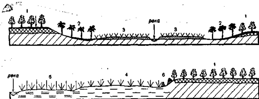
Рис. 63. Схема распределения почв и растительности по рельефу в Замбии (по М. Коул, 1963):
