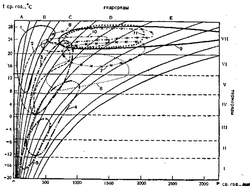
Рис. 14. Климатические ареалы основных почвенных типов мира в гидротермической системе координат (по В. Р. Волобуеву, 1963);
