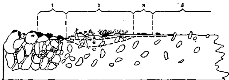
Рис. 55. Полигональная каменная арктическая тундра. Гренландия (по Уголини, 1966):
