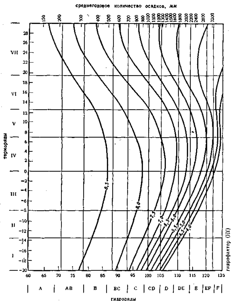
Рис. 5. Значение pH в слое 0—20 см в главных типах почв мира в связи с гидротермическими условиями (по В. Р. Волобуеву, 1963)
