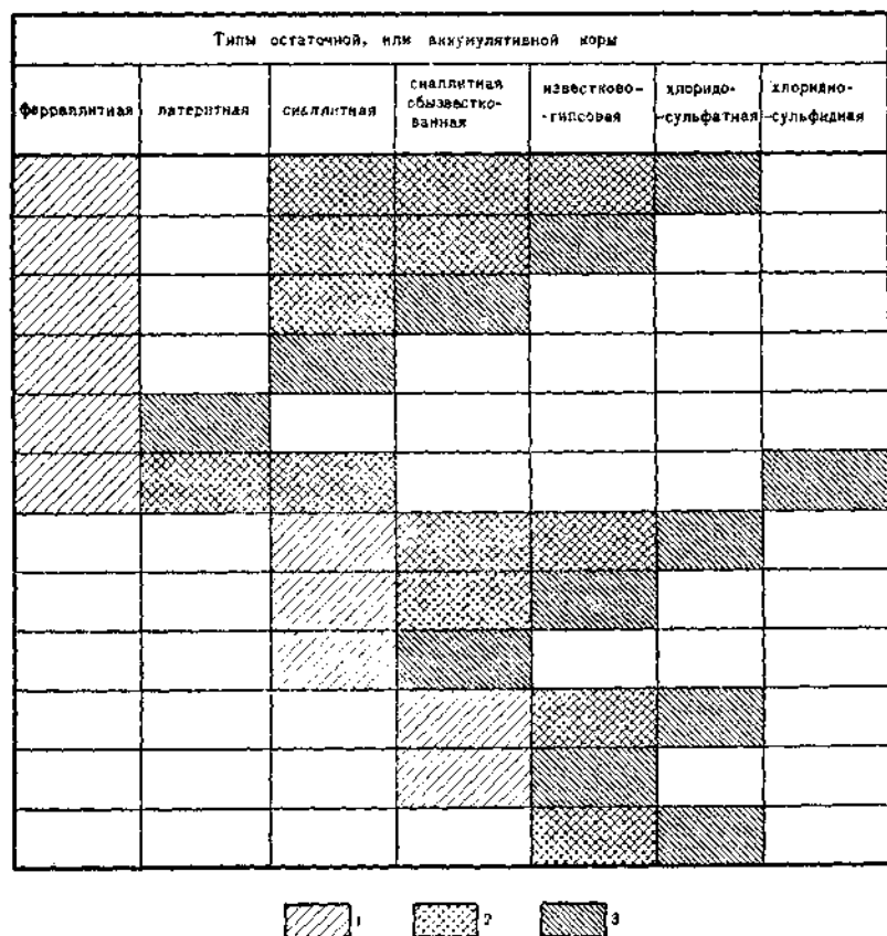
Рис. 14. Типы сочетаний остаточных (1), транзитных аккумулятивных (2) и аккумулятивных (3) кор выветривания
