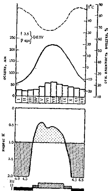
Рис. 44. Гидротермические условия в районах распространения серых лесных почв. Усл. знаки см. рис. 36
