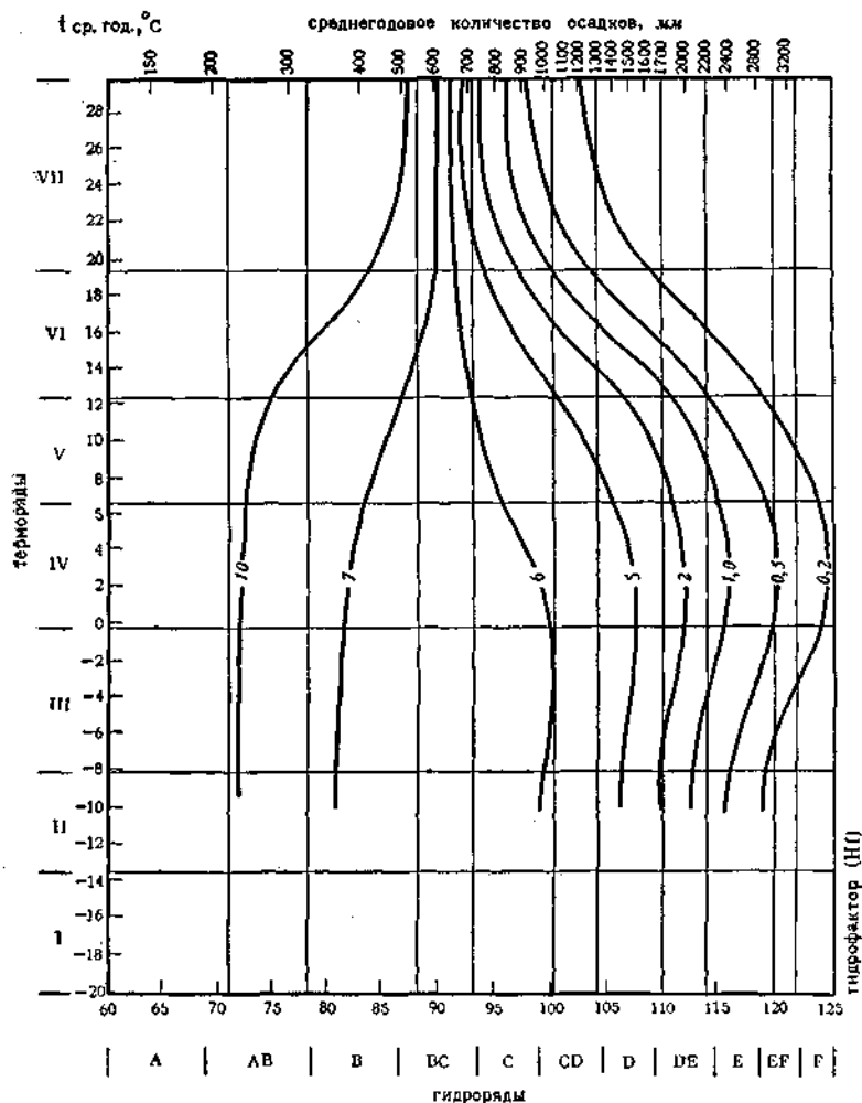
Рис. 6. Содержание карбонатов ( \% \text{CO}_2 ) в верхнем метровом слое почв в связи с гидротермическими условиями (по В. Р. Волобуеву, 1963)
