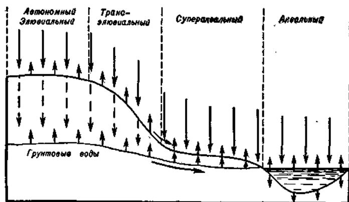
Рис. 20. Схема элементарных ландшафтов, по Б. Е. Полюнову
