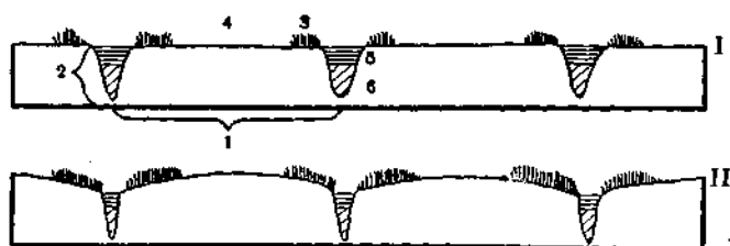
Рис. 29. Микрорельеф и почвы вершин увалов арктической тундры на о-ве Большом Ляховском (по Н. А. Караваевой, 1969):
