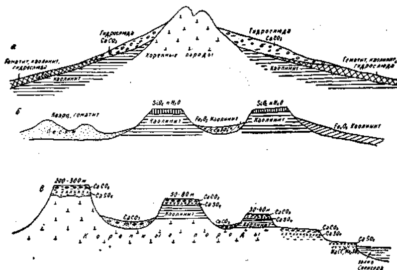
Рис. 68. Схематические профили распределения ландшафтно-геохимических реликтов:
