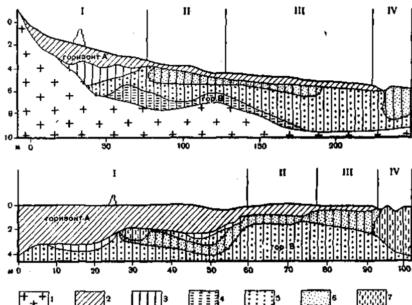
Рис. 62. Почвенно-геохимическая catena в бассейне оз. Чад (по Бокье, 1970).
