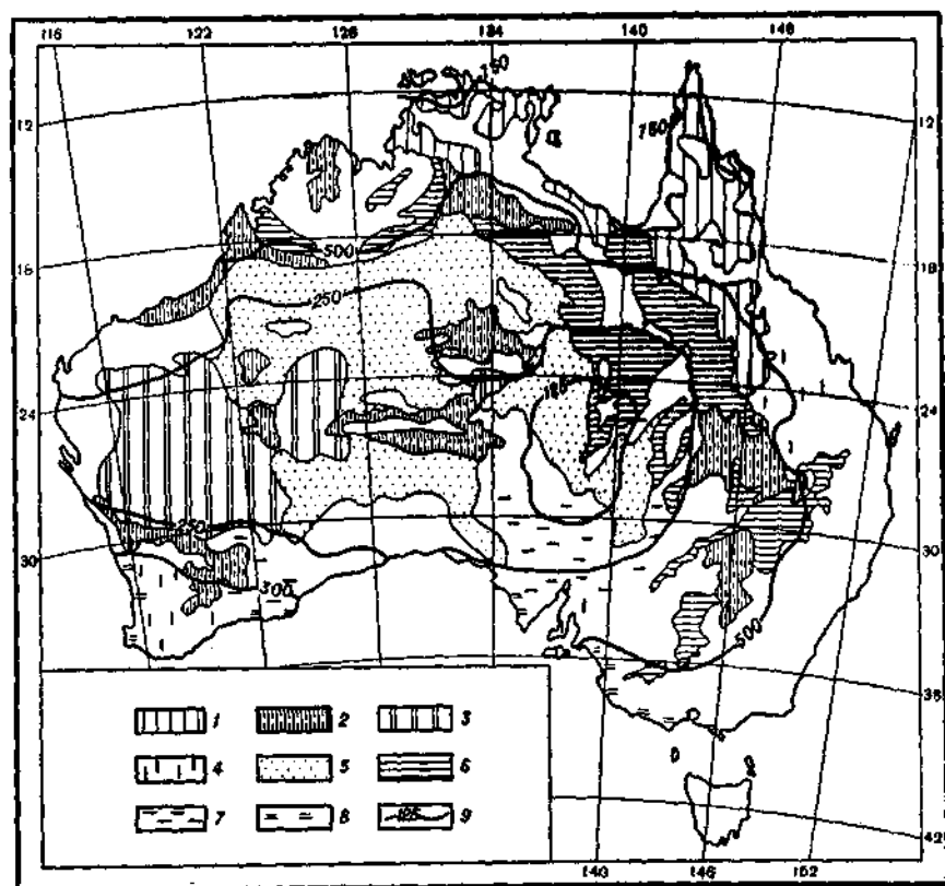
Рис. 64. Ландшафтно-геохимические реликты Австралии. Реликты древних элювиальных и супераккумуляных влажнотропических ландшафтов. Области распространения древней каолинит-гематитовой (латеритной) коры выветривания:
