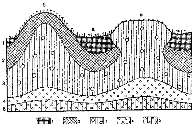
Рис. 31. Схема почвенного комплекса на гряде, на полуострове П'ягина (по Е. Н. Наумову, 1965):
