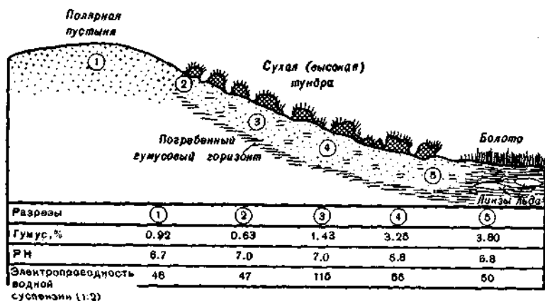
Рис. 28. Сочетание почв по рельефу в арктических полярных пустынях. О. Принс-Патрик (Tedrow, 1968)
