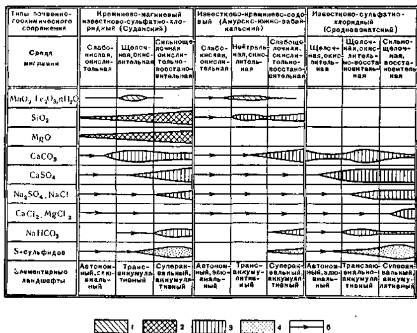
Рис. 22. Типы почвенно-геохимических сопряжений семиаридных и аридных областей.
