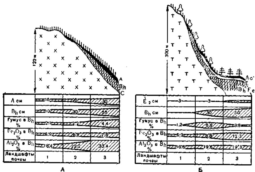
Рис. 23. Почвенно-геохимические сопряжения холодных гумидных областей северной Норвегии (по М. А. Глазовской, 1968):
