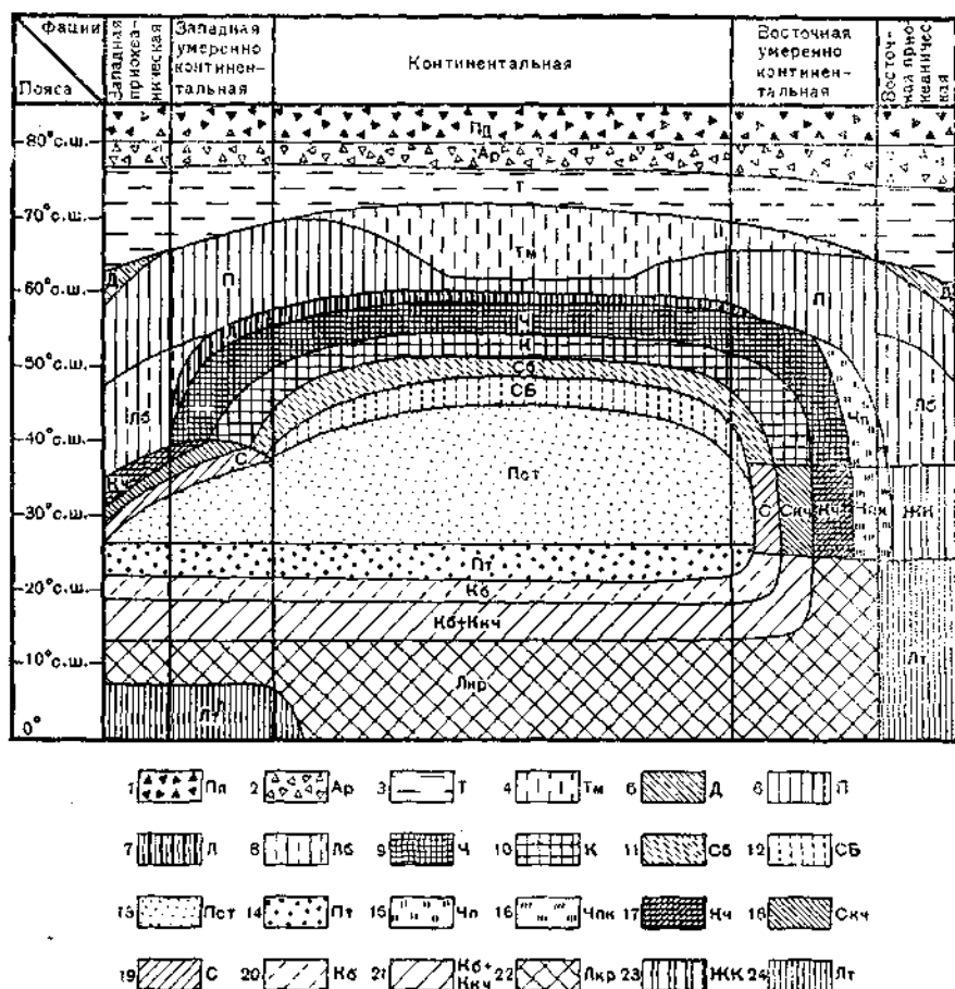
Рис. 12. Схема горизонтальных почвенных зон северного полушария на «идеальном континенте».
