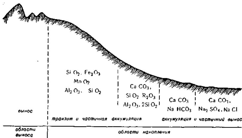
Рис. 48. Схема распространения продуктов выветривания и почвообразования в Маньчжурии и Монголии (по В. А. Ковде, 1969)
