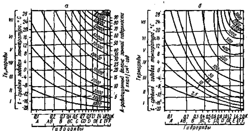
Рис. 2. Затраты энергии в почвообразовании ( \text{кал}/\text{см}^2 \cdot \text{год} ): а — суммарные затраты энергии в биогеоценозе на почвообразование; б — запасы энергии, накапливаемые в годичном приросте растительной массы, надземной и корневой (по В. Р. Волобуеву, 1963)
