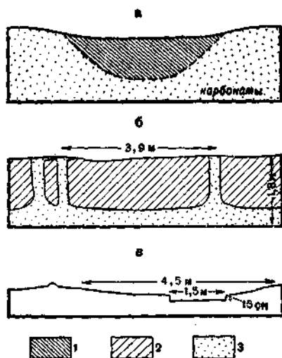
Рис. 66. Разрезы через комплексы «гильган»:
