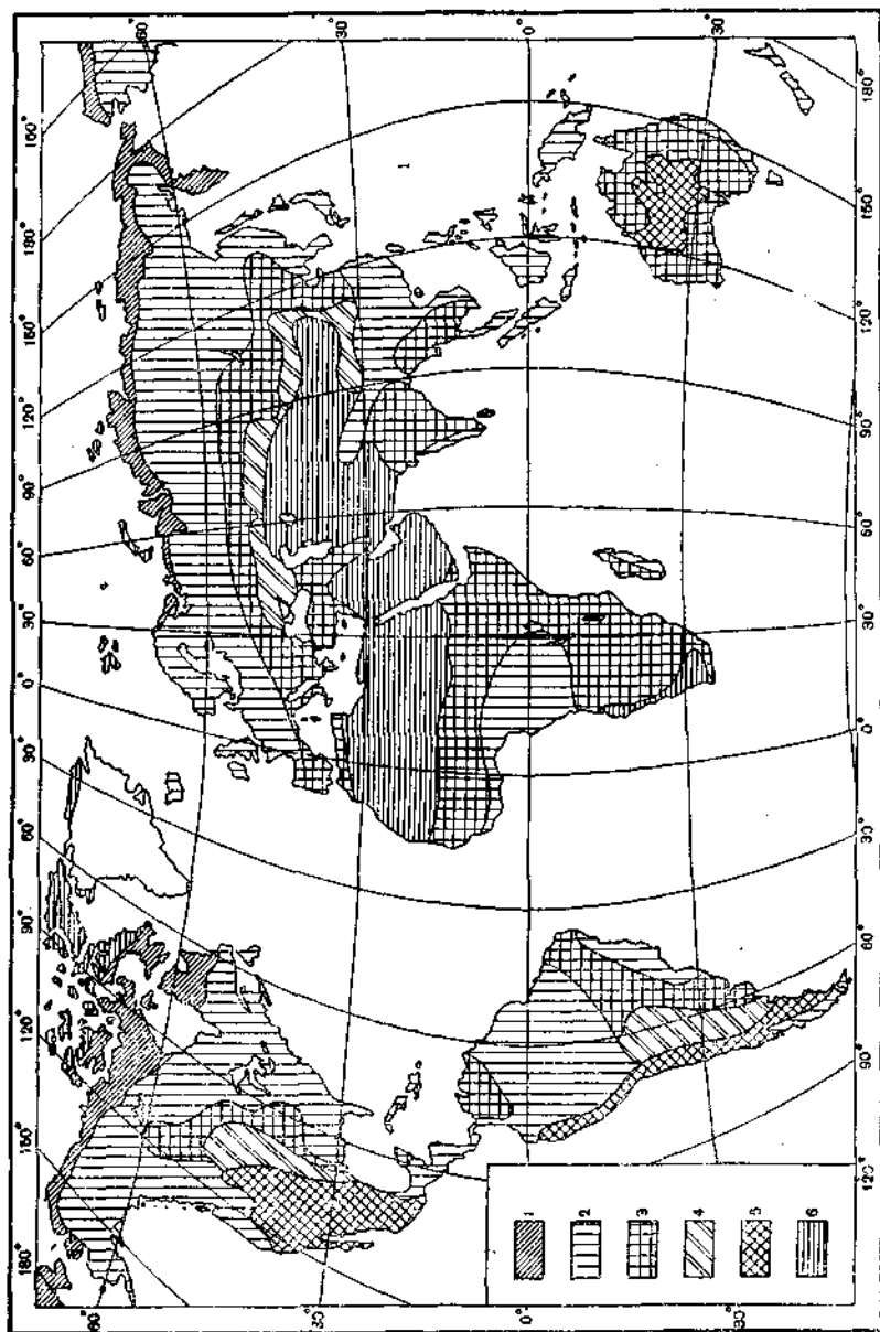
Рис. 3. Почвенно-геохимические поля.
