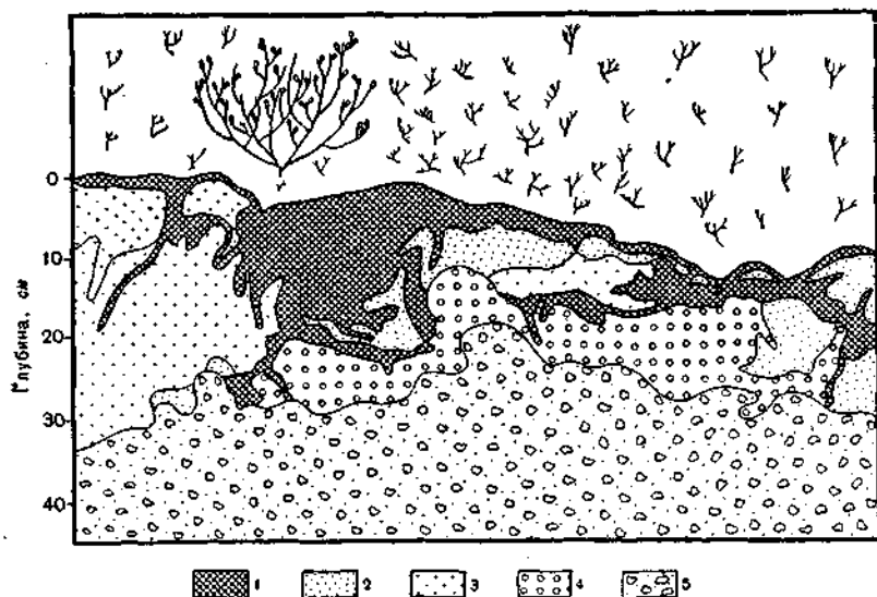
Рис. 56. Криотурбация в арктотундровых почвах. Гренландия (по Уголини, 1966):
