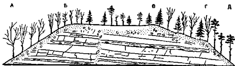
Рис. 38. Схематический профиль распределения растительности и почв в Средне-Германских горах на пестроцветных песчаниках.
