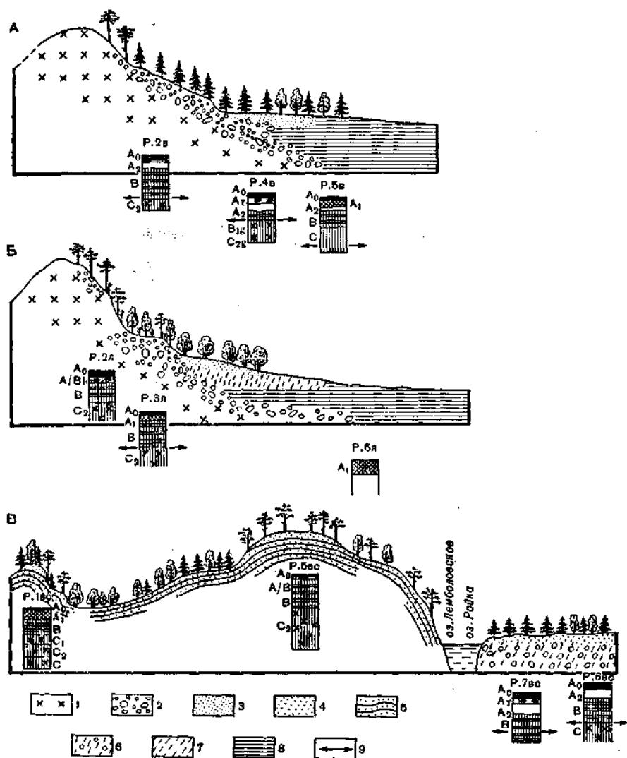
Рис. 34. Распределение почв по рельефу в южной Карелии (по Т. А. Рожновой, 1963):
