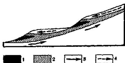
Рис. 60. Схема процесса денудации лесных почв на склонах после порубки лесов (Оберу и Миньену): 1 — латерит; 2 — латеритизованная кора выветривания; 3 — направления движения; 4 — направления движения поверхностных склоновых вод
