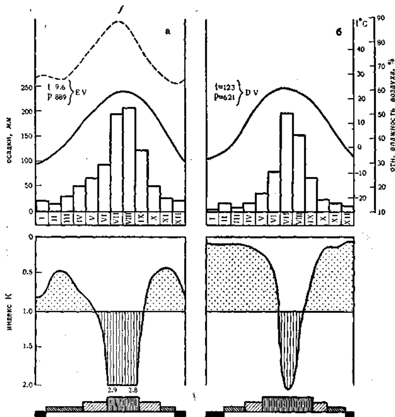
Рис. 39. Гидротермические условия в районах распространения: а — бурых лесных почв Дальнего Востока, б — коричневых почв Китая (б). Усл. знаки см. рис. 36
