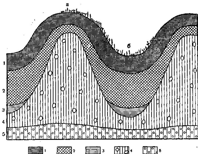
Рис. 32. Схема почвенного комплекса в ложине на п-ове Пьягина (по Е. Н. Наумову, 1965):
