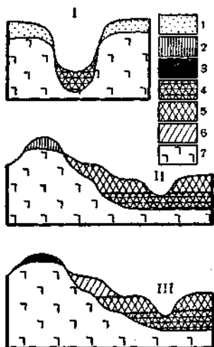
Рис. 15. Сопряженные остаточные и аккумулятивные коры выветривания в области развития изверженных пород (по Б. Б. Полюнову, 1956):
