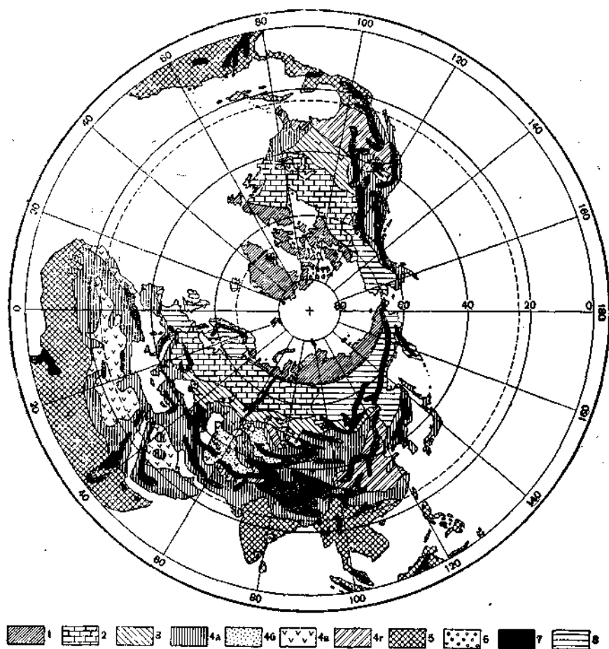
Рис. 1. Почвенные зоны Северного полушария (схема) (В. В. Докучаев, 1899): 1 — бореальная (арктическая); 2 — лесная; 3 — черноземных степей; 4 — азральная (а — каменная, б — песчаная, в — солончаковая, г — лессовая); 5 — латеритные почвы; 6 — аллювий; 7 — горные цепи; 8 — облесенные территории
