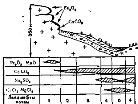
Рис. 25. Почвенно-геохимическое сопряжение высокогорных пустынь Центрального Тянь-Шаня (по М. А. Глазовской, 1968):
