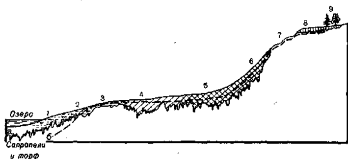
Рис. 35. Схема расположения растительности и почв по профилю в аласе (по В. А. Шелудяковой и др., 1954):
