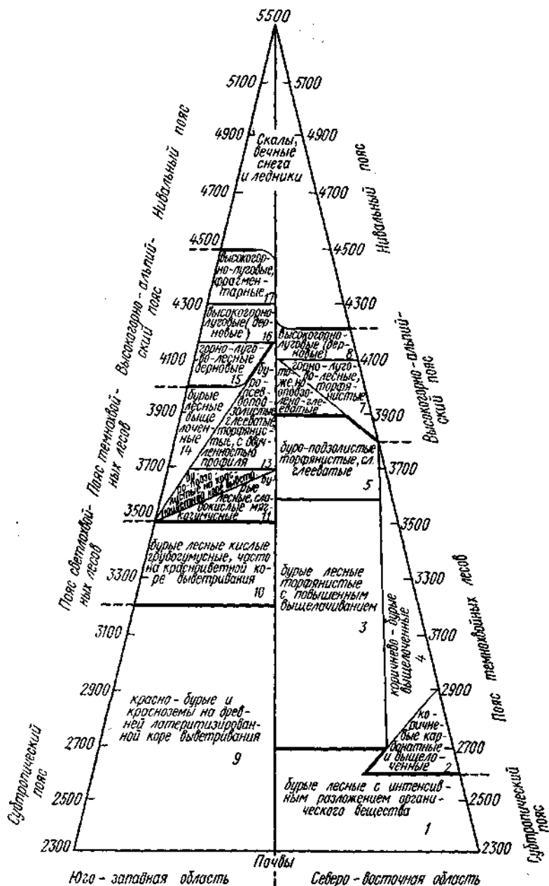
Рис. 54. Схема вертикально-поясного распределения растительности и почв в Восточном Тибете (по С. В. Зоняну, 1964)
