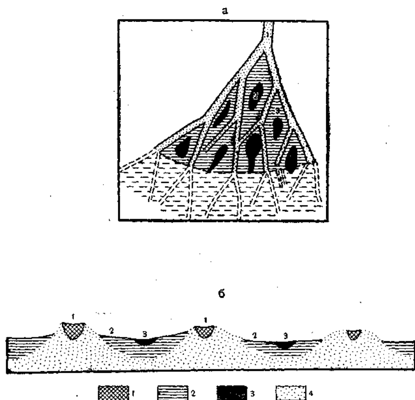
Рис. 40. Схема отложений и профиля дельты Хуанхэ (по В. А. Ковда, 1964):
