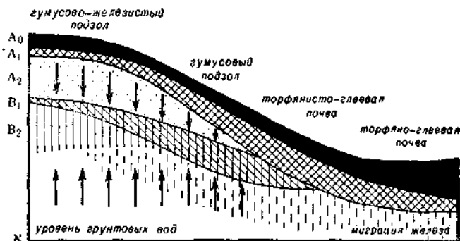
Рис. 37. Почвенная catena на склоне песчаного холма при близком стоянии грунтовых вод в ландшафтах в Гасконии (по Дюшофуру, 1948)
