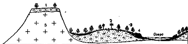
Рис. 33. Распределение почв по элементам мезорельефа в предтундровых редколесьях Северной Лапландии (по М. А. Глазовской, 1964): 1 — полигональные комплексы карликовых железистых подзолов и маломощных каменистых почв; 2 — карликовые иллювиально-железисто-гумусовые подзолы под березовыми редколесьями; 3 — торфянистые иллювиально-гумусовые подзолы; 4 — торфяно-глеевые почвы
