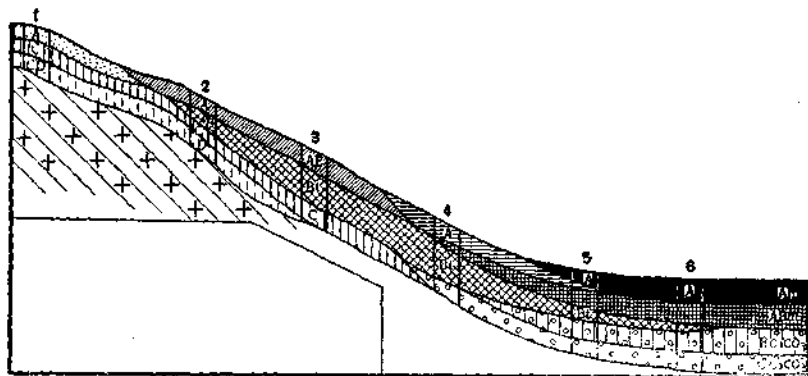
Рис. 42. Распределение почв по рельефу Гранитного массива в Болгарии (по В. Койкову и др., 1969):
