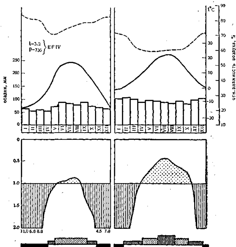
Рис. 57. Гидротермические условия в районах распространения дерново-подзолистых и бурых лесных почв Северной Америки. Усл. знаки см. рис. 36
