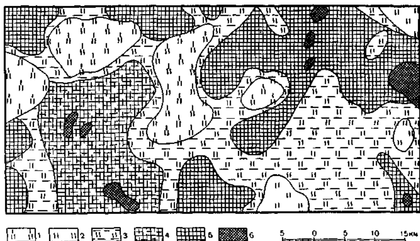
Рис. 51. План лугово-степного комплекса с суффузионным макрорельефом в Прикаспии (по Е. Н. Ивановой и др.):
