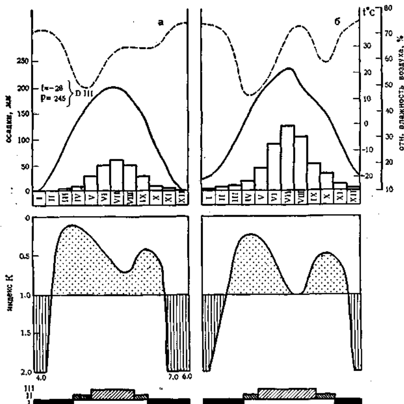
Рис. 47. Гидротермические условия в районах распространения: а — черноземов в Монголии; б — черноземовидных почв прерий в Маньчжурии. Усл. знаки см. рис. 36
