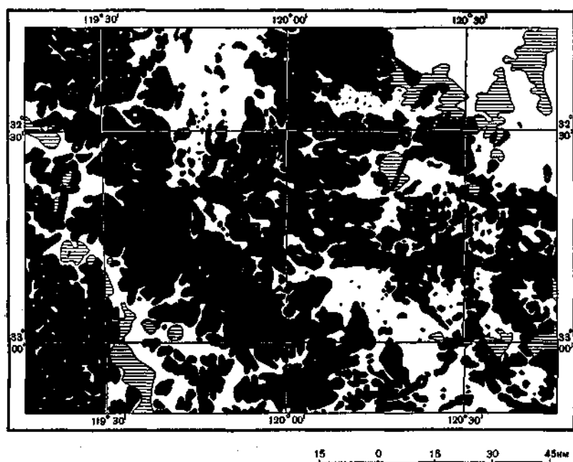
Рис. 65. Карта части Западной Австралии между оз. Кинг и хр. Бремера. Черный цвет — поверхность пенеплена с сохранившейся латеритной корой; белый — склоны, где латеритная кора смыта; штриховка — озера
