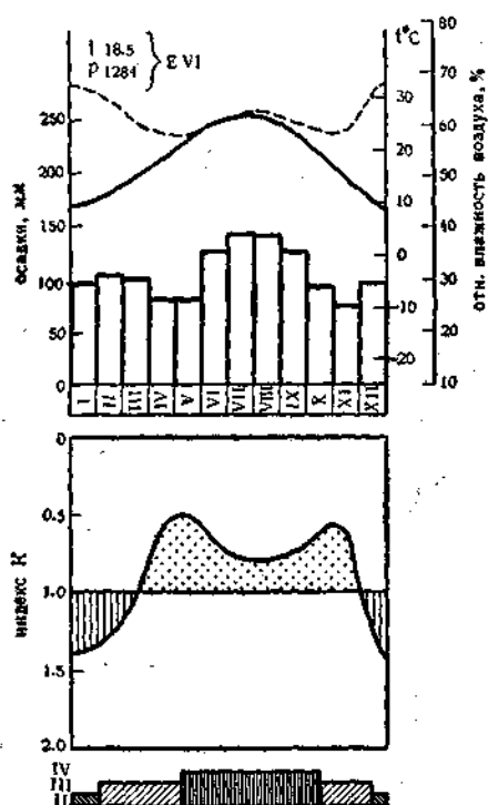
Рис. 58. Гидротермические условия районов распространения желтоземов и красноземов в США. Усл. знаки см. рис. 36
