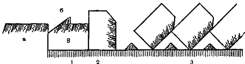
Рис. 160. Схема положения пластов при вспашке винтовым плугом со скимкольтером: 1 — положение пласта после последовательного прохода ножа (а) скимкольтера (б) и лемеха корпуса (в); 2 — положение пласта после прохода отвала корпуса; 3 — окончательное положение пластов.
