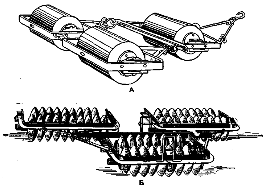
Рис. 185. Гладкий каток, применяемый для весеннего укатывания травяного поля лугового севооборота (А) и глыбодроб (Б), применявшийся при вспашке плугом без предплужника и для ломки ледяной корки на озимых.
