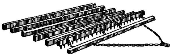
Рис. 180. Гвоздевка (по Азребаев).
