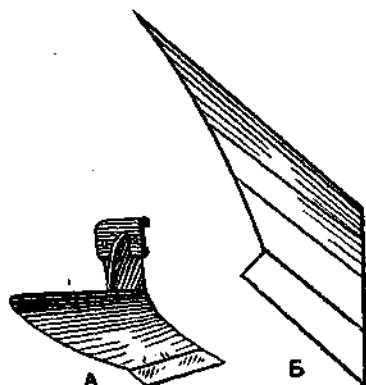
Рис. 163. Цилиндрический отвал: А — вид сбоку; В — проекция.
