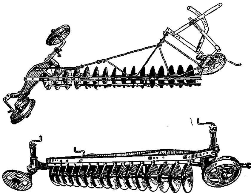
Р и с. 186. Тракторный «пшеничный плуг», марка ППТЗ, применяемый исключительно для лущения жнивья.
