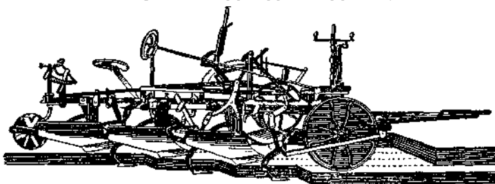
Рис. 181. Трехкорпусный тракторный плуг с предплужниками и почвоуглубителями в каждой борозде.
