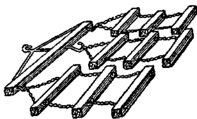
Рис. 178. Схема устройства волокуши.
