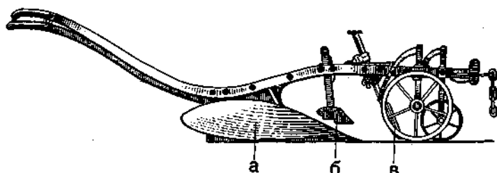
Рис. 159. Однокорпусный английский плуг с укороченным винтовым отвалом (среднего типа). Впереди главного корпуса (а) помещается скимкольтер (б) и перед ним нож (в).
