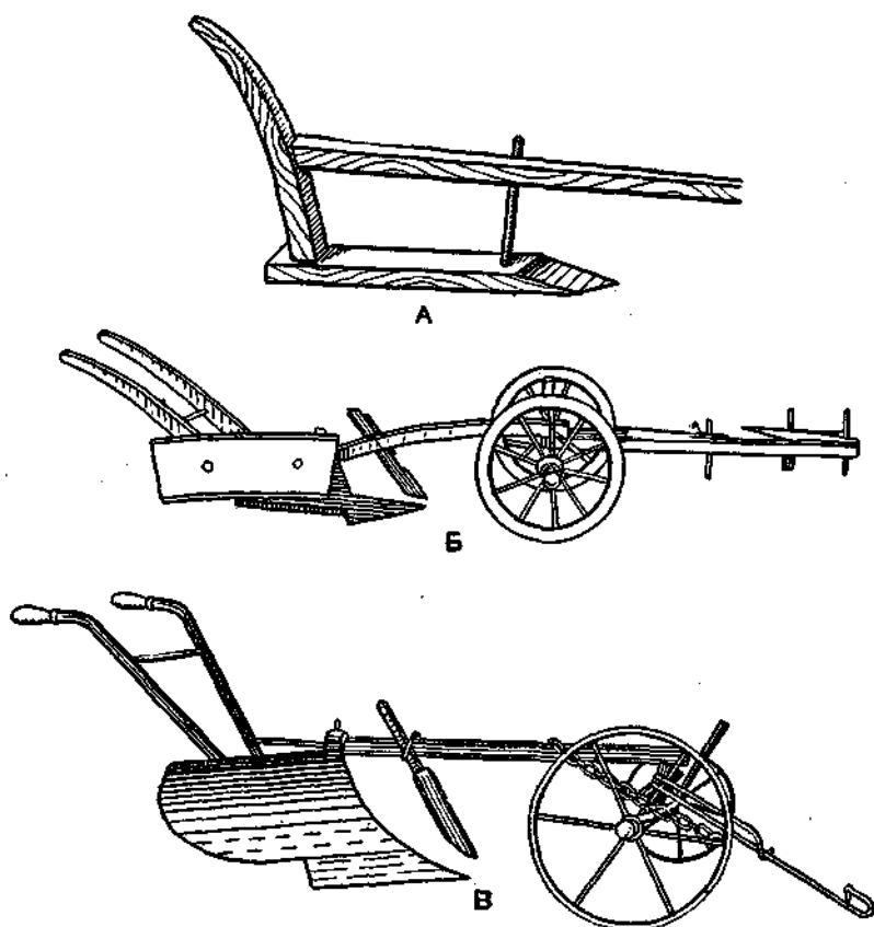
Р и с. 152. Прimitивные орудия обработки почвы, применявшиеся на Украине и в б. Новороссии: А — рало; Б — малороссийский сабан, развившийся из двух соединенных рал; В — стальная копия сабана завода Рансома — «Новороссийский колонийский плуг».
