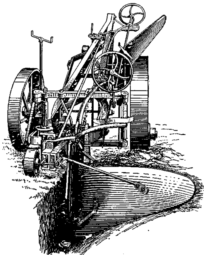
Рис. 177. Райольный плуг.
