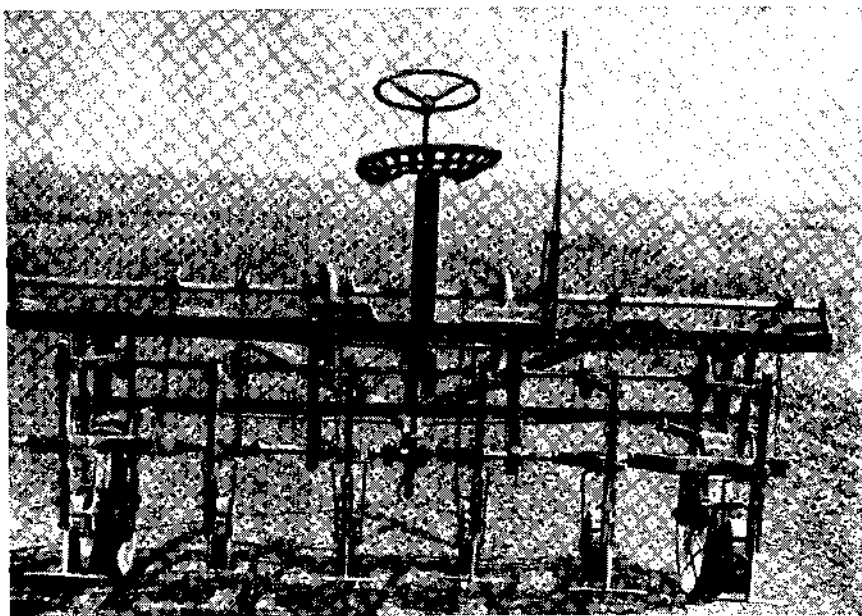
Рис. 190. Экстирпатор тов. Кастрного (слесарь совхоза им. Сталина, Воронежской обл.).
