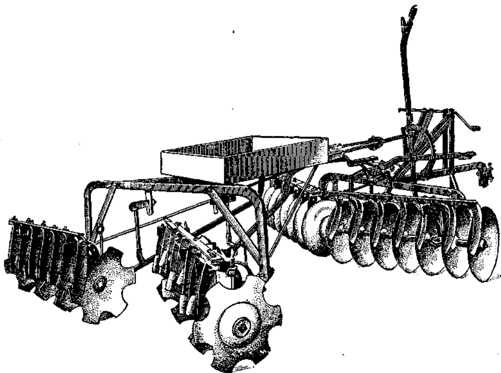
Рис. 196. Дисковый культиватор, вынужденно применяемый при неглубокой обработке долговременных лугов американскими плугами.
