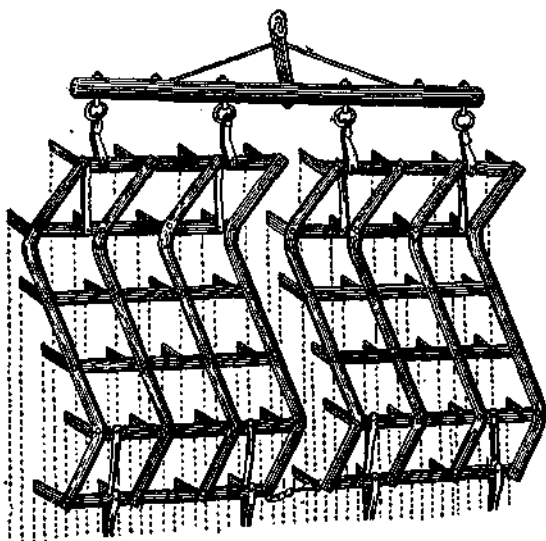
Р и с. 156. Два звена современной тяжелой бороны.
